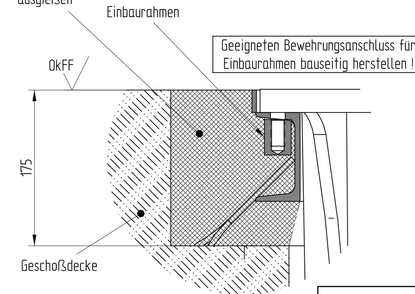
EINZELHEIT B
