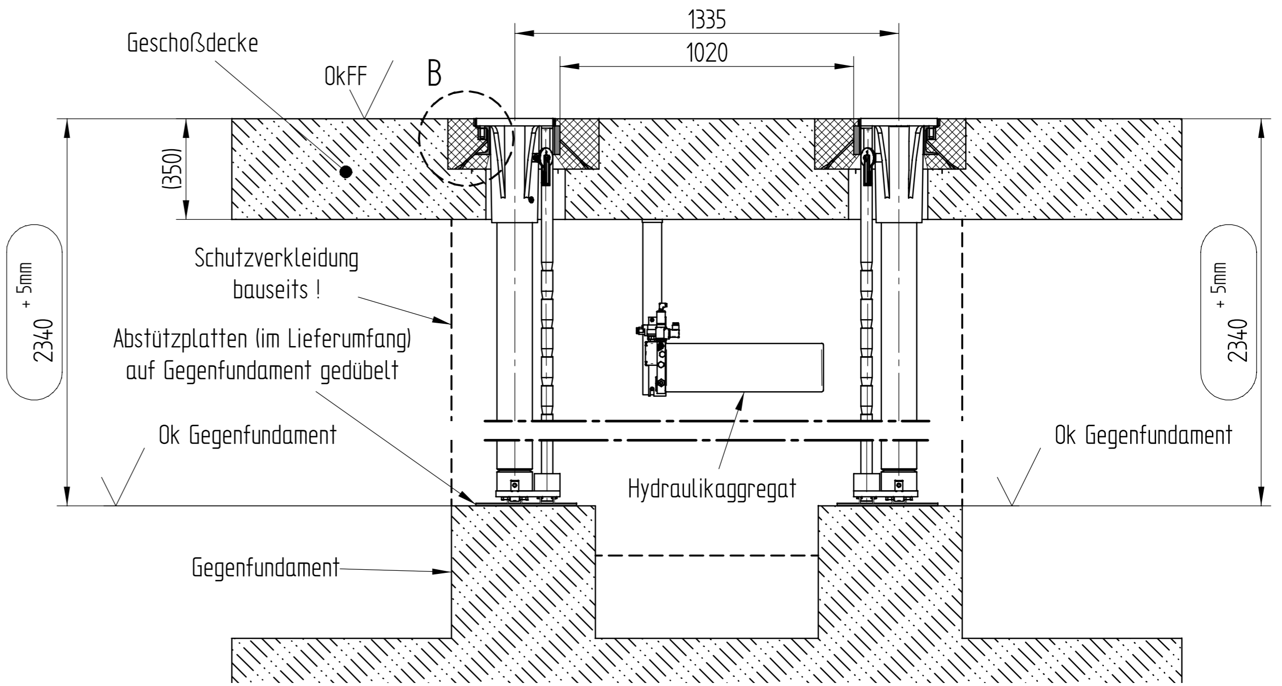
SCHNITT A-A
